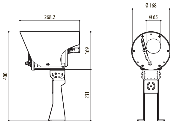
Рис. 46 NVX, крепление к парапету.
