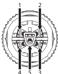
Abb. 20 Vorderansicht der Pins und Innenansicht der Klemmen.
