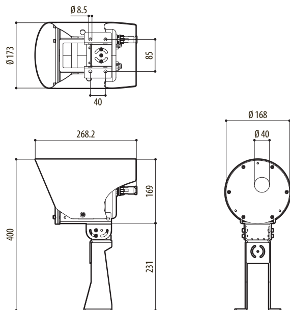
Рис. 49 NTX, крепление к parapety.
