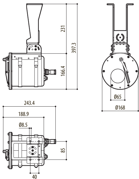
Abb. 47 NVX, deckenbefestigung.
