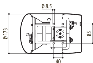
Abb. 45 NVX, Wandbefestigung.
