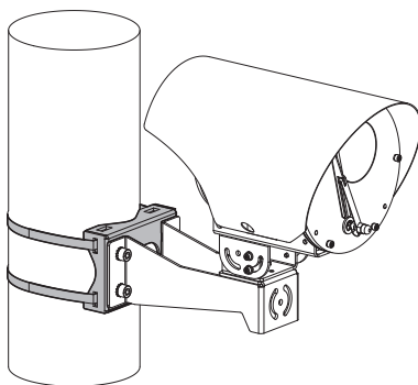
Рис. 38 UEAP.
