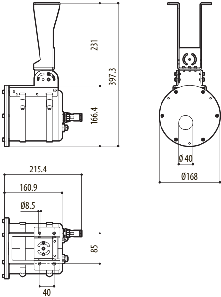
Fig. 50 NTX, fixation au plafond.
