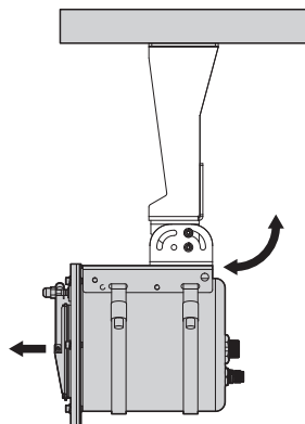
Fig. 15 Esempio di installazione a soffitto, rotazione verticale, 0°.
