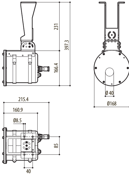
Abb. 50 NTX, deckenbefestigung.
