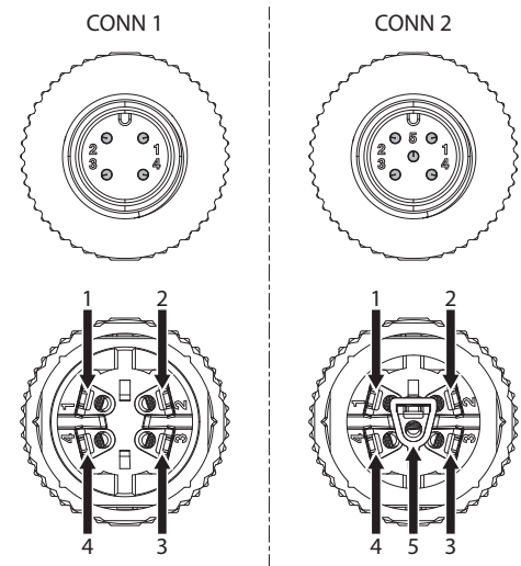
Рис. 20 Вид контактов спереди и вид клемм изнутри.
