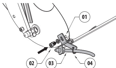
Abb. 36 GEKO IRH.
