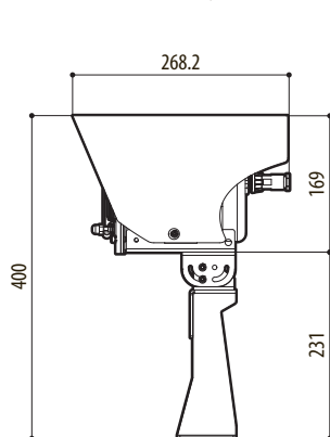
Fig. 46 NVX, fissaggio a parapetto.
