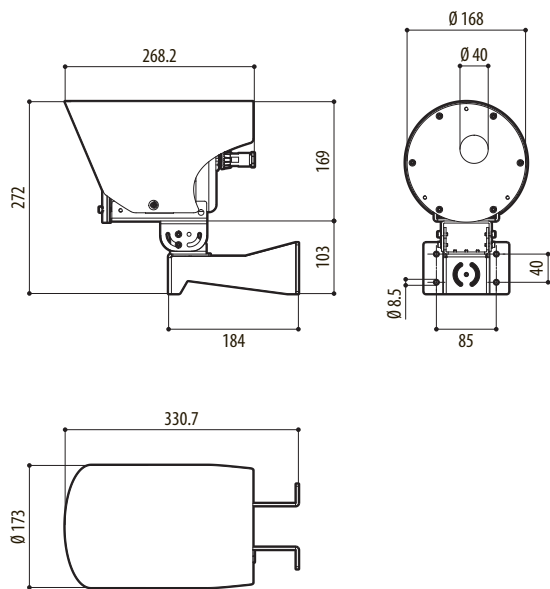
Abb. 48 NTX, Wandbefestigung.
