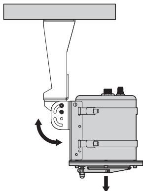
Abb. 16 Beispiel Deckenmontage, Vertikale Drehung, -90°.
