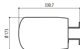
Abb. 45 NVX, Wandbefestigung.
