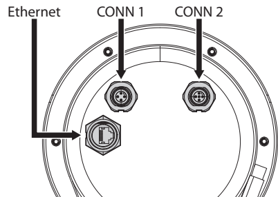
Abb. 19 Rückansicht der Kamera. Steckverbinder von der Kameraseite.
