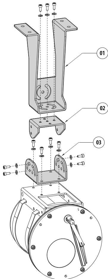
Abb. 10 Deckenbefestigung.
