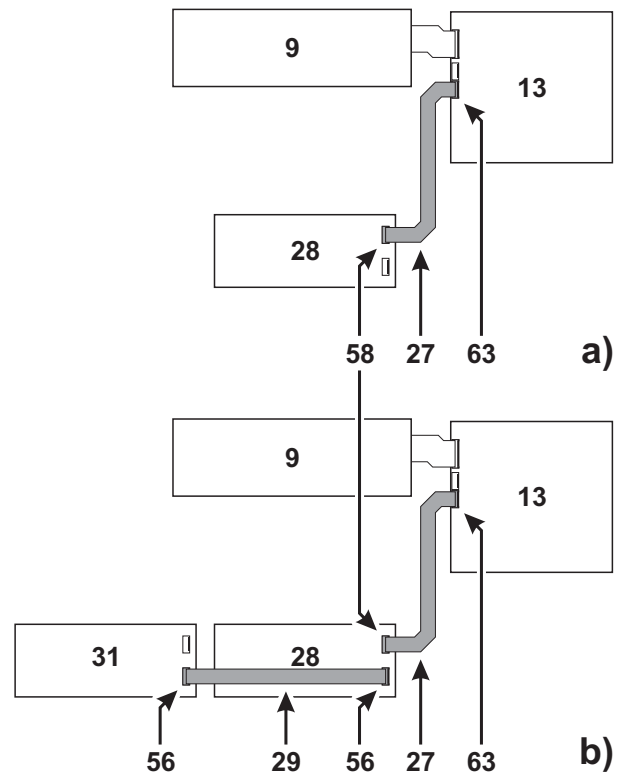
Figura 9 Conexión de UN Módulo de Extinción (a) o DOS Módulos de Extinción (b) a la Central J424: 9) Placa de Control Principal; 13) Placa Principal; 27) y 29) cable plano para conectar los Módulos de Extinción; 28) Módulo de Extinción n.º. 1; 31) Módulo de Extinción n.º. 2; 56) Conector para el Módulo de Extinción consecutivo 58) Terminal para conectar a la Placa Principal; 63) Conector para el Módulo de Extinción n.º. 1.
