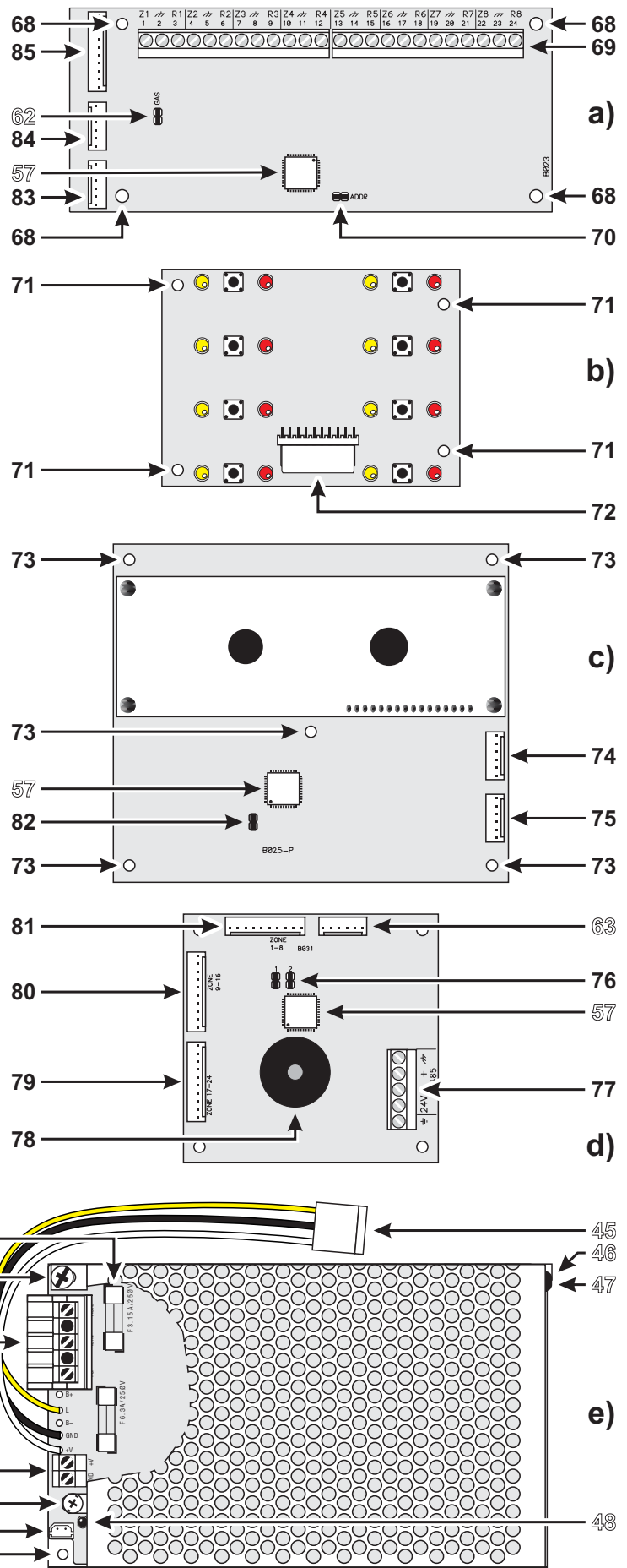
Figura 6 Identificación de las Partes: a) Módulo Expansor; b) Tarjeta de Control del Expansor; c) Módulo Display; d) Interface del Repetidor RS485; e) Fuente de Alimentación de la Central J424
