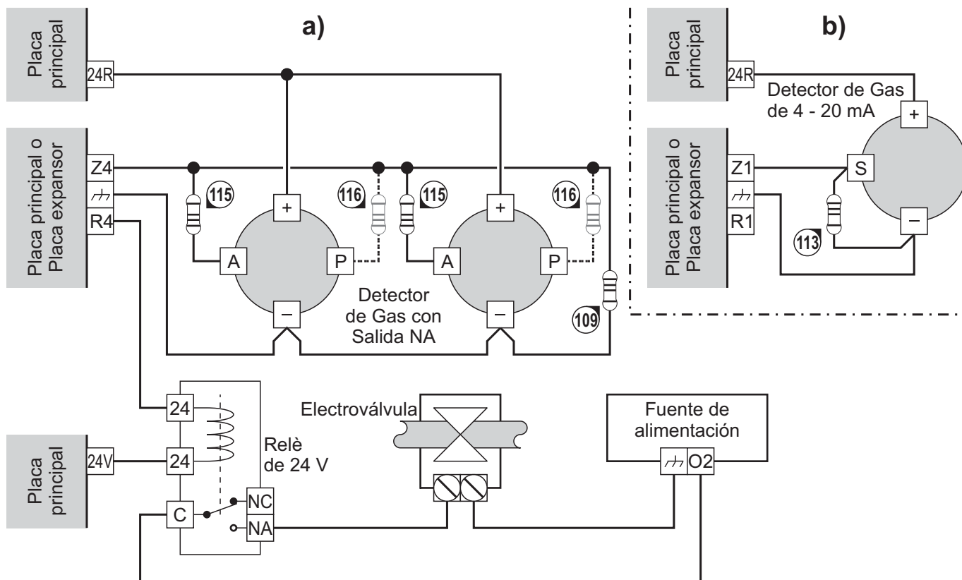
Figura 16 Conexión de un detector de Gas con Salida Normalmente Abierta (a) y un detector de Gas de 4 - 20 mA (b): 109 Resist. Fin de Línea de 3900 ohm, 1/4 W (naranja-blanco-rojo-oro); 111 Resist. de 680 ohm; 113 Resistencia de 470 ohm, 2 W; 115 Resistencia de 680 ohm si la opción "Detector de Gas NA x 2" está deshabilitada o de 820 ohm si está habilitada; 116 Resistencia de 820 ohm a conectar sólo si la opción "Detector de Gas NA x 2" está habilitada.
