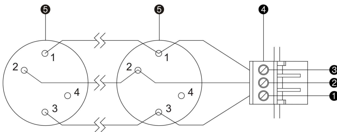
Figura 4: conexión de la línea de zona de los detectores CCO-170
