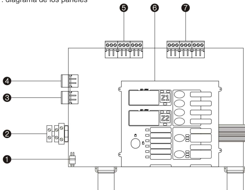
Figura 1: diagrama de los paneles
