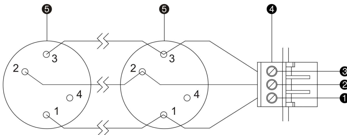
Figura 5: conexión de la línea de zona de los detectores CCO-300
