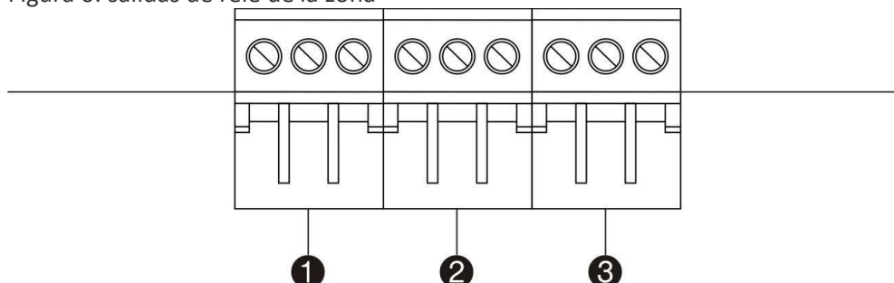
Figura 6: salidas de relé de la zona
