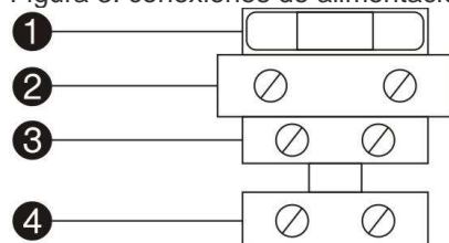
Figura 3: conexiones de alimentación eléctrica
