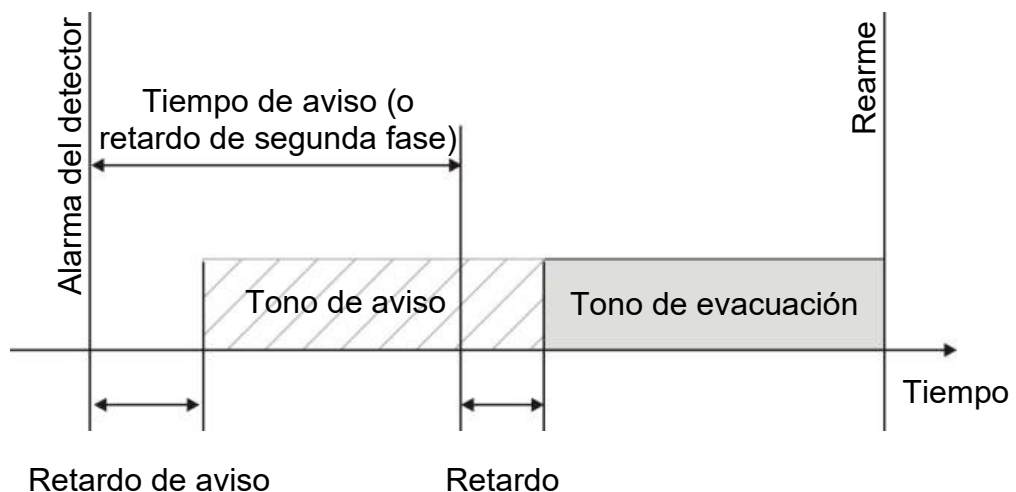
Figura 26: Alarma del detector con retardo de segunda fase
