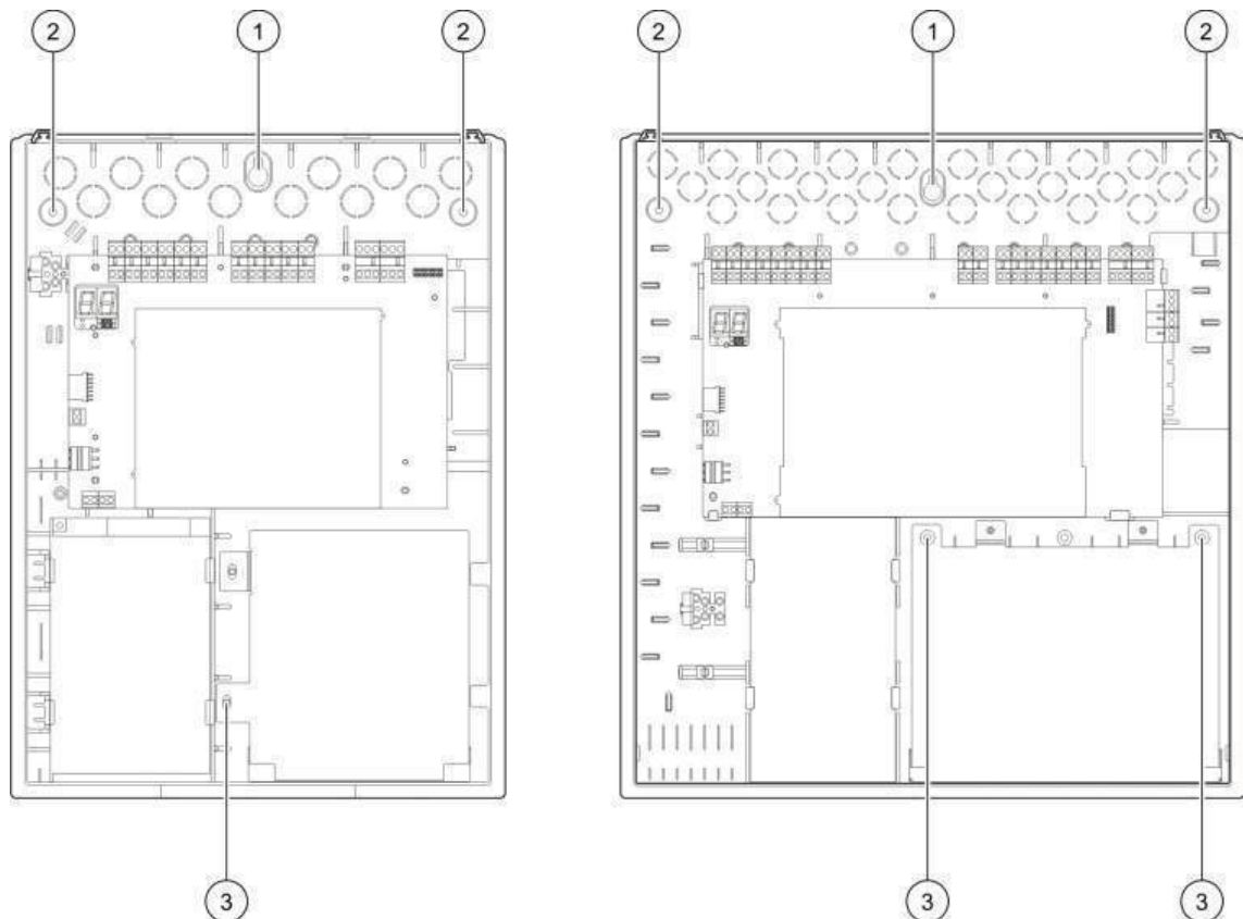
Figura 3: Ubicaciones de los orificios de montaje
