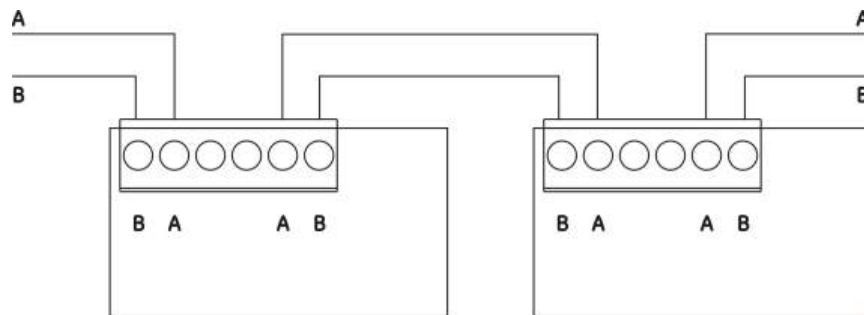
Figura 13: Conexiones de la tarjeta de red
