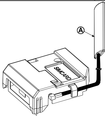
A. External GSM antenna Fig. 3 Optional external GSM antenna
