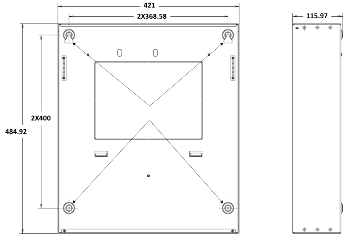
Figura 6: Detalles de las medidas del alojamiento
