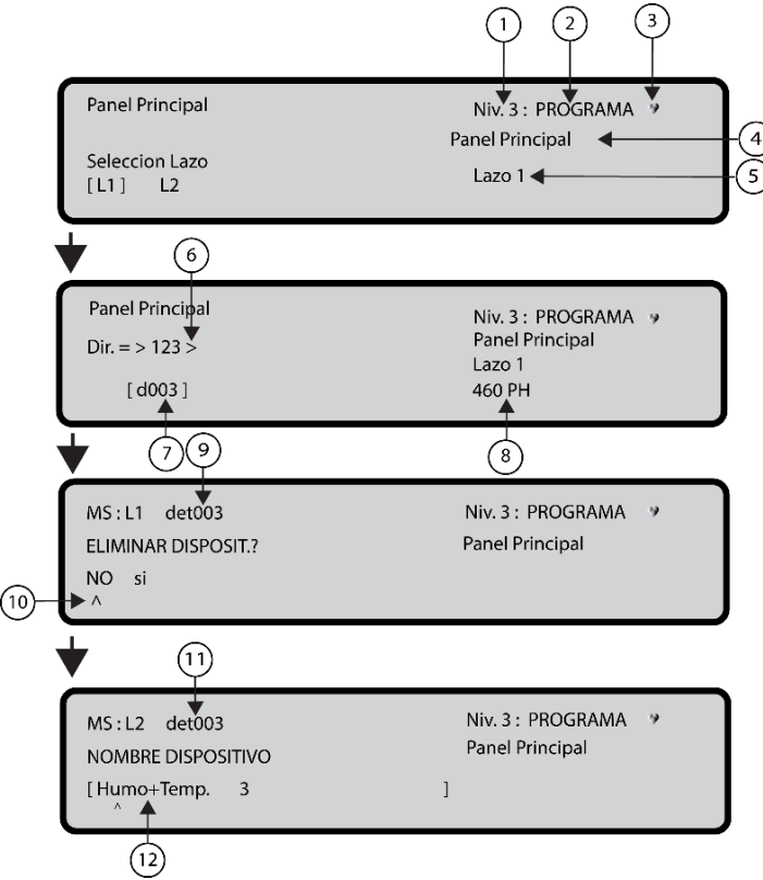
Figura 25: Selección y programación de dispositivos en el lazo
