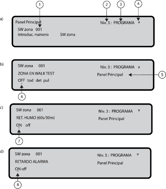
Figura 27: Programación de la verificación de alarma del detector de retardo de opción
