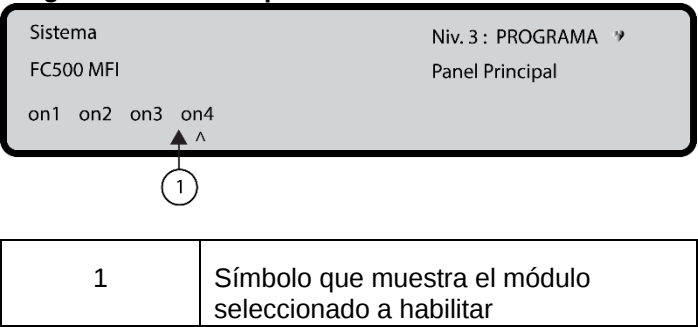
Figura 30: Pantalla para habilitar el módulo FC500MFI
