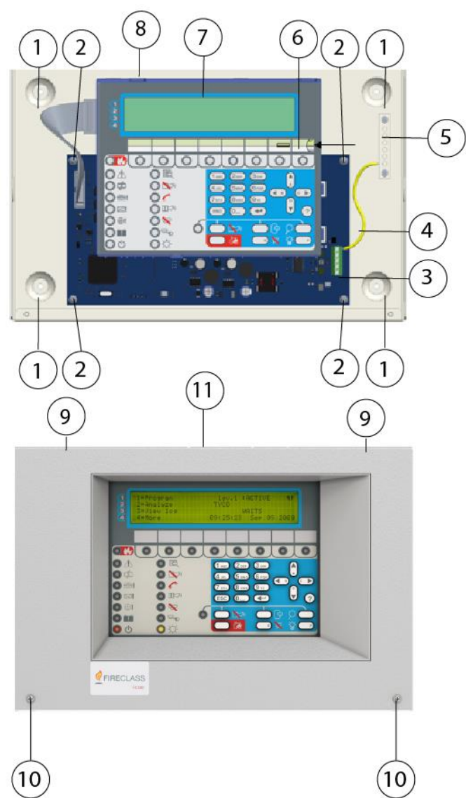
Figura 7: Instalación del repetidor FC500
