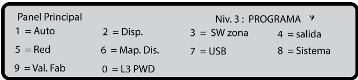
Figura 21: Pantalla PROGRAMAR
