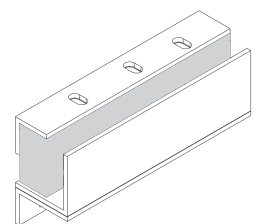
PERFIL 'ZL' 'ZL' PROFILE
