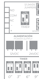
CABLEADO WIRING
