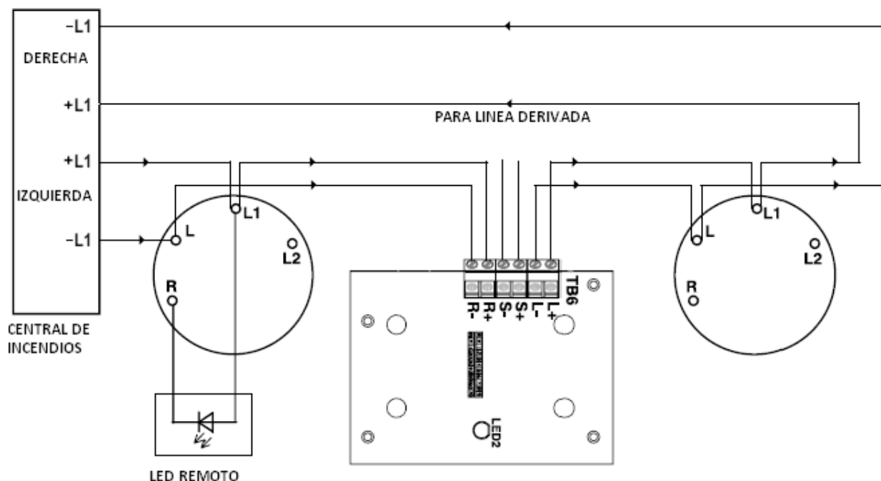
Figura 4: FC410LI. Diagrama simplificado de cableado.
