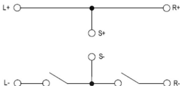
Figura 1: FC410LI Esquema de operación
