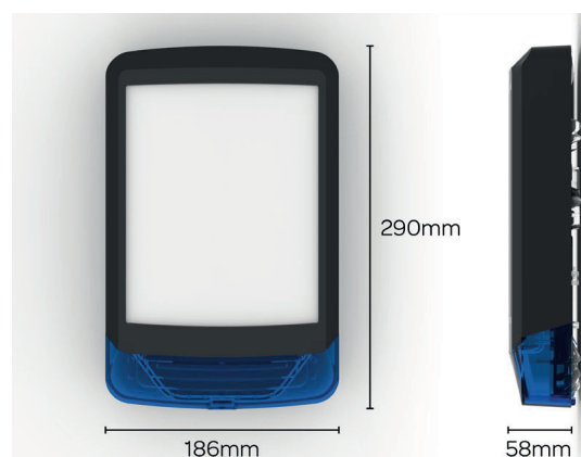
DIMENSIONES DE LA TAPA ALTRA-SOUNDCOVER-X1
